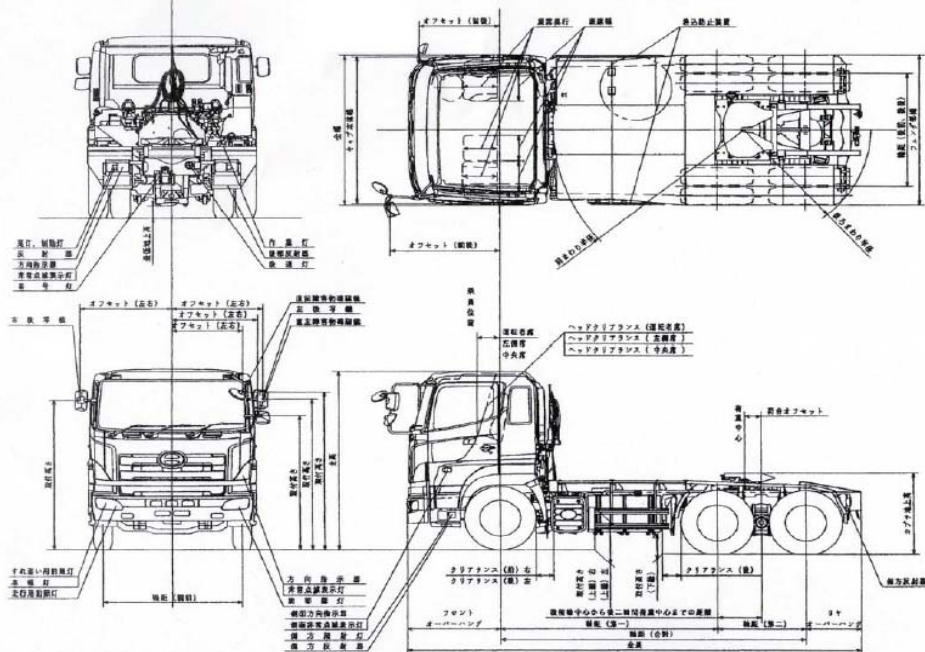
4-1 外觀四面圖
